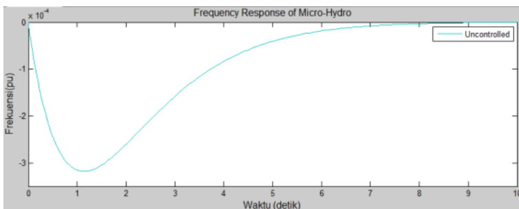
Gambar 3. Simulasi pembangkit mikrohidro tanpa kontrol
