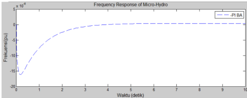
Gambar 4. Simulasi pembangkit mikrohidro dengan PI-BA
