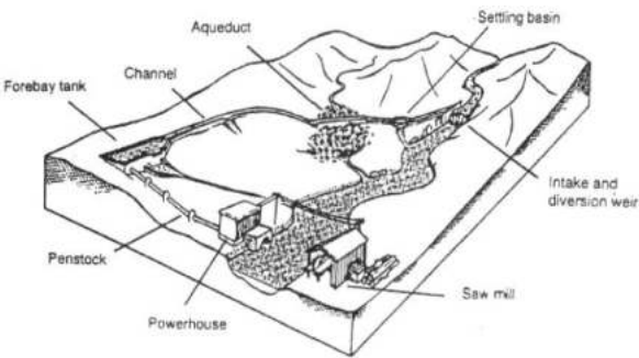
Gambar 2.1 Komponen utama skema mikrohidro
