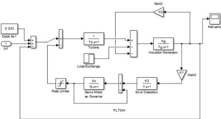
Gambar 1. Pemodelan pembangkit mikrohidro
