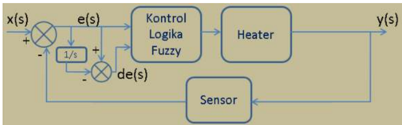
Sistem Kontrol Close Loop Pengaturan Suhu menggunakan Kontroler Fuzzy
