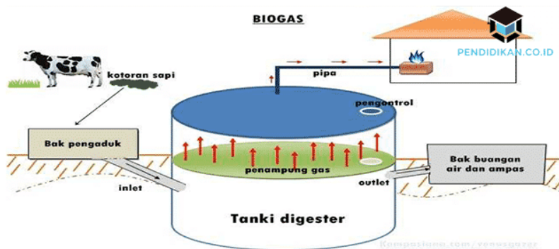
Gamabr 1. Proses Terbentuknya Biogas
