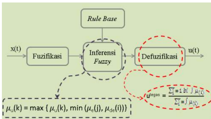
Perancangan Kontroler Fuzzy yang digunakan
