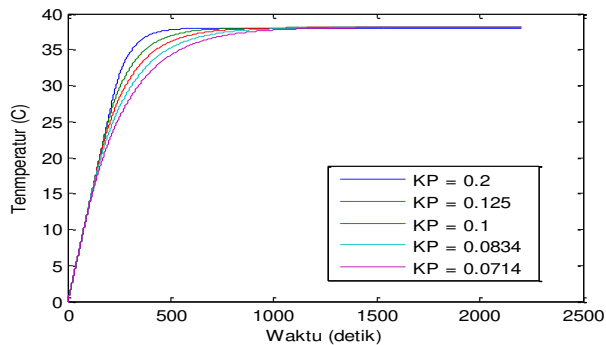
Output Suhu dari Kontroler Fuzzy dengan Gain Kp yang disesuaikan
