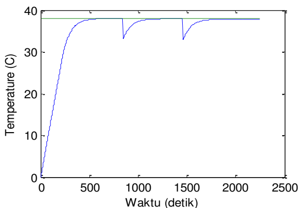
Output kontroler Fuzzy ketika diberi beban/gangguan
