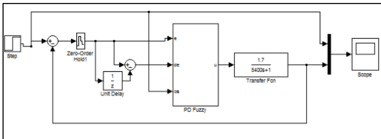
Simulasi Simulink Kontroler Fuzzy
