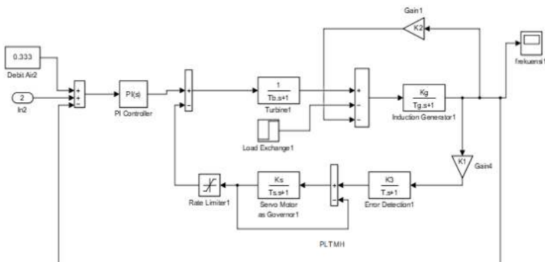
Gambar 2. Pemodelan pembangkit mikrohidro dengan kontrolller PI
