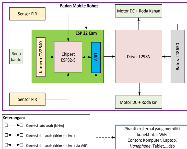
Konfigurasi pembangunan mobile robot
