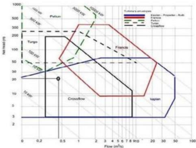
Gambar 2.2 Grafik Pemilihan Turbin
